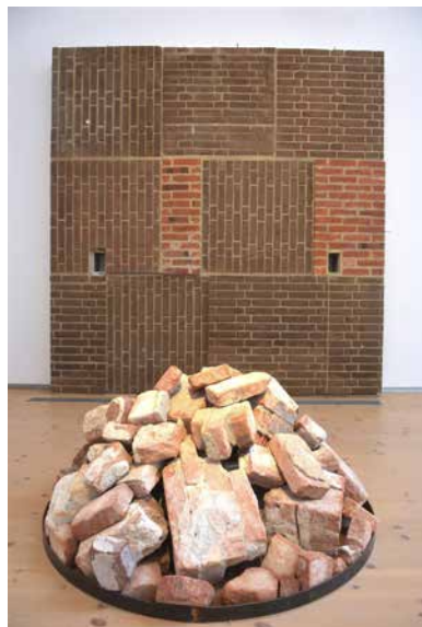
Tegel satt med cementbruk går inte att separera, men kan återvinnas i utsågade block.
